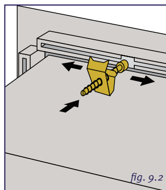
Bottom view of sink / Vue du dessous de l'évier
